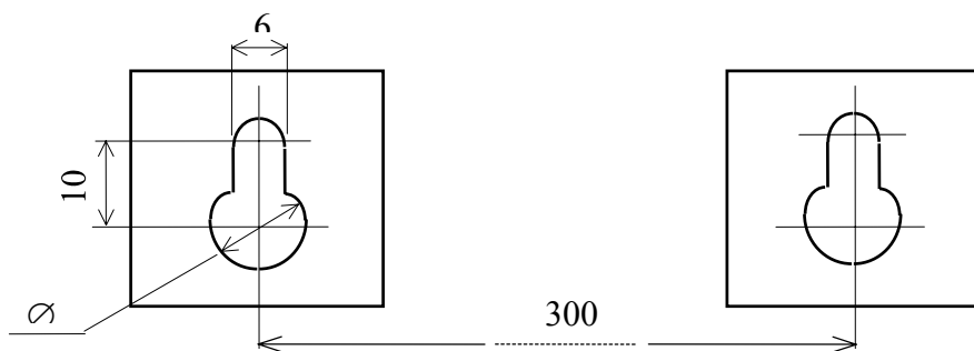
Рисунок 3.1 - Разметка крепления прибора БЛ-40М на стене
