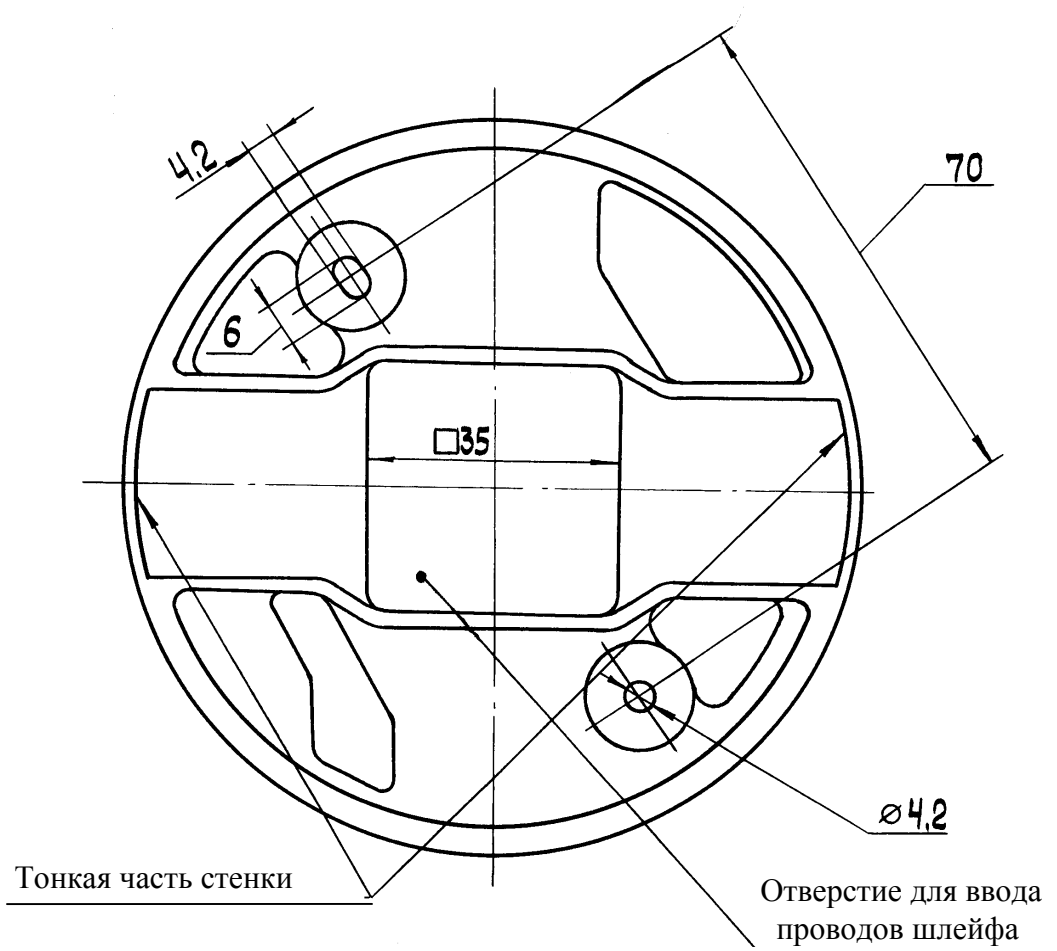
Рисунок 5 - Вид розетки со стороны контактов
