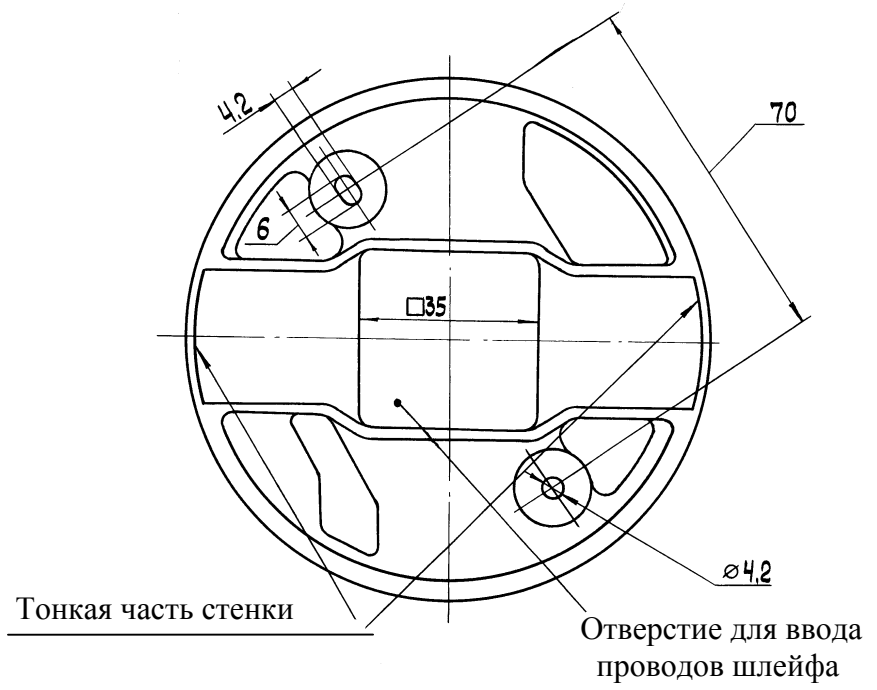
Рисунок 5 - Установочные размеры розетки
