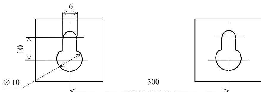
Рисунок 4 - Разметка крепления прибора ППК-2М на стене
